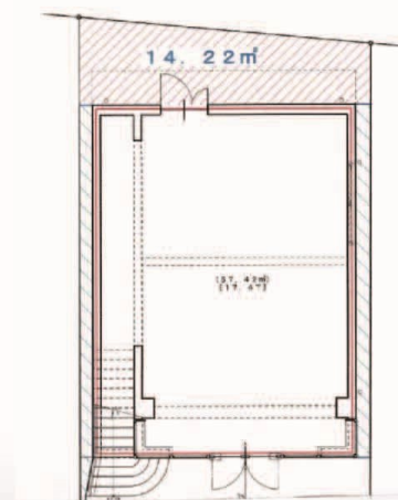
間取図
