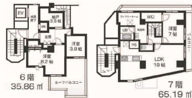
間取図
