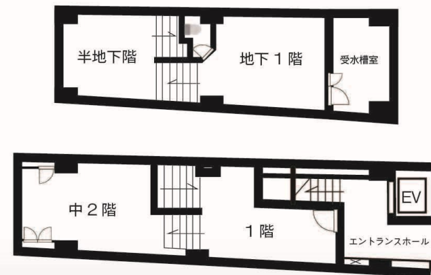
間取図
