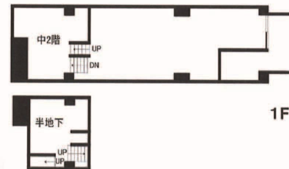
間取図
